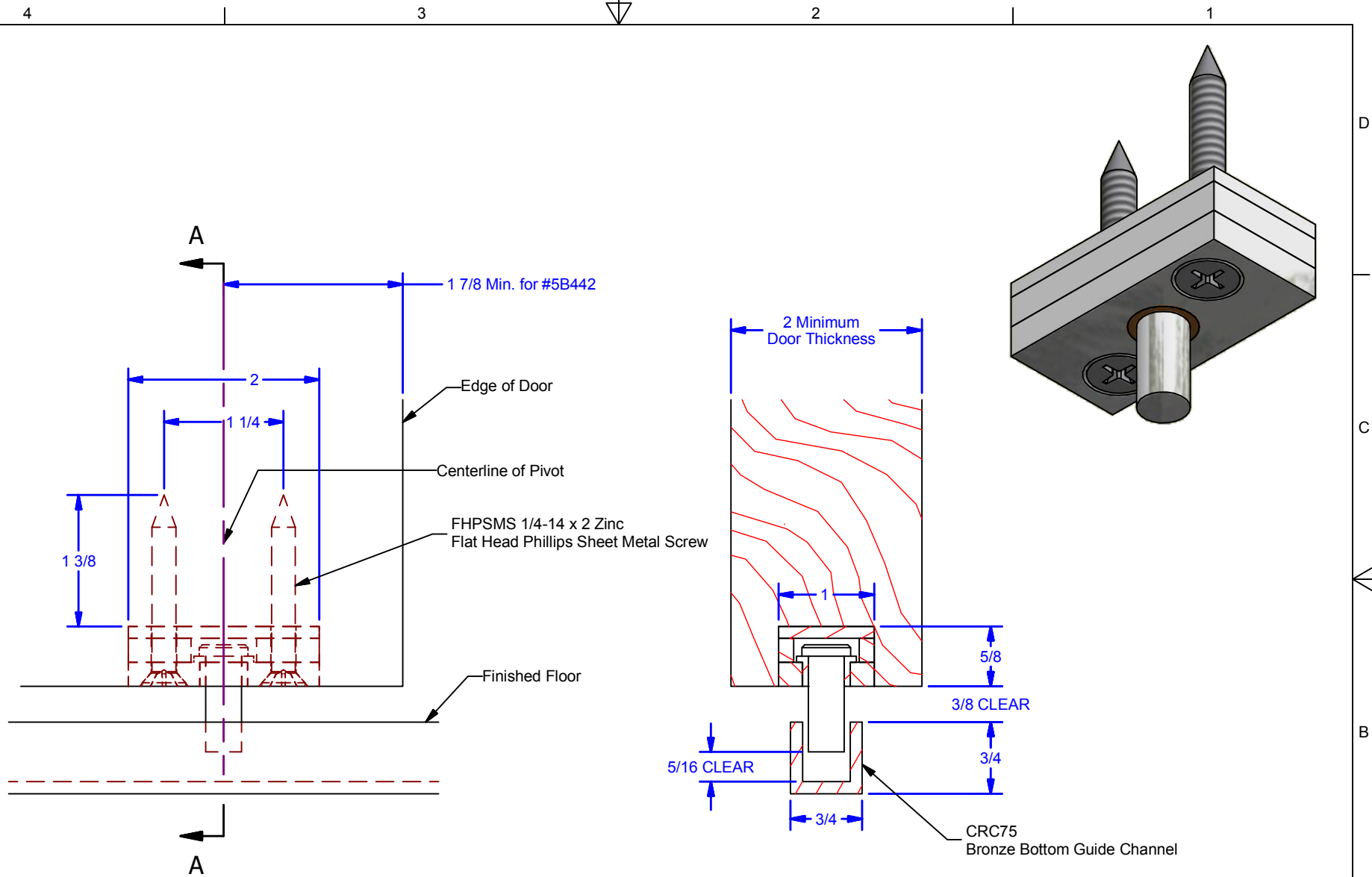
SECTION A-A
